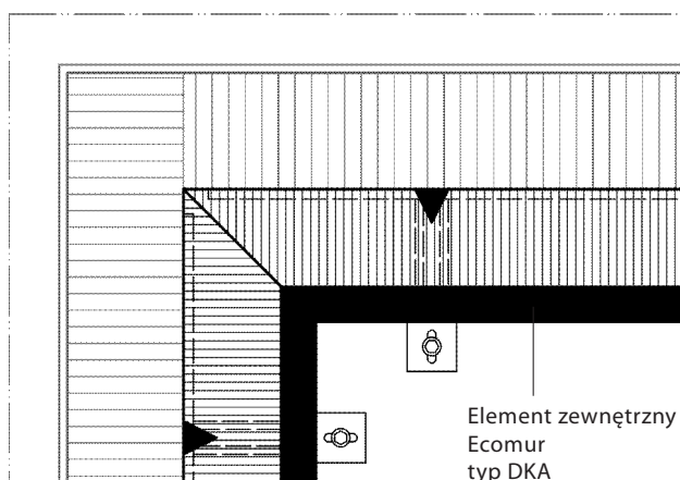
Narożnik zewnętrzny Przekrój poziomy
