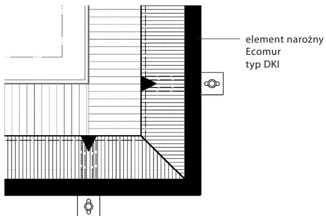
Narożnik wewnętrzny Przekrój poziomy
