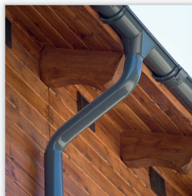
Ruukki, System rynnowy – 125 mm lub 150 mm. Komponuje się idealnie z blachodachówką, blachą na rąbek stojący, blachą trapezową. System składa się z: zaślepek, rynny, narożnika zewnętrznego, łącznika rynnowego, haka rynnowego, wylotu, narożnika wewnętrznego, kolana, obejm, obejm rury spustowej, wylotu rury. Wykończenie powierzchni: powłoka Pural. Kolory: ciemnozielony, biały, grafitowy, czerwony, ciemnobrązowy, czarny, ceglasty, czekoladowobrązowy. Gwarancja: 20 lat.
