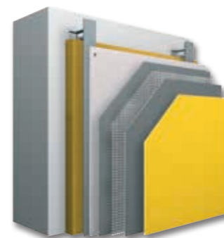
System StoVentec - bezspoinowy
