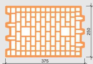
Przekrój pustaka Porotherm 25 E3
