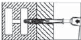
2 Osadź kotwę
