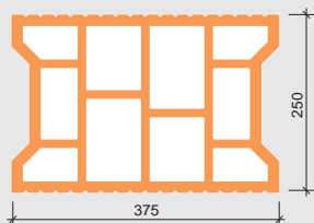
Przekrój pustaka Porotherm 25 AKU
