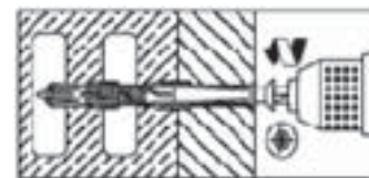
3 Wkręć wkręt w tuleję kotwy
