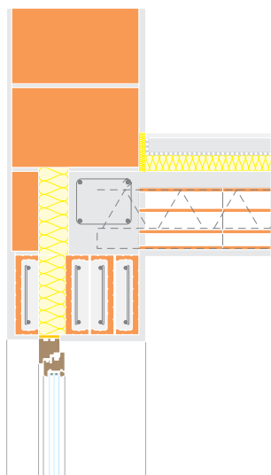
ściana Porotherm 44 P+W / EKO+ / Profi / Dryfix
