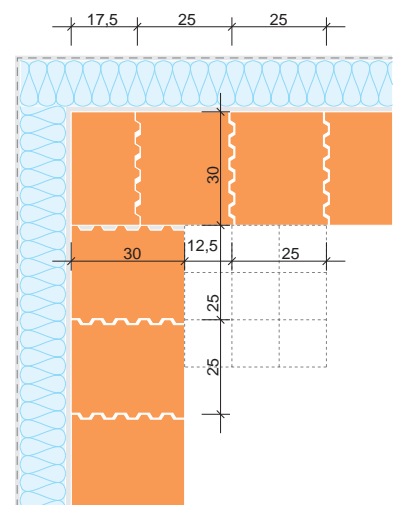
rysunek drugiej warstwy
