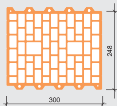
Przekrój pustaka Porotherm 30 E3
