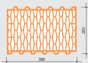
Schemat narożnika
