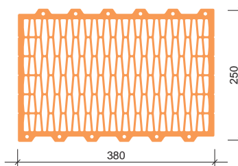
Porotherm 38 Si
