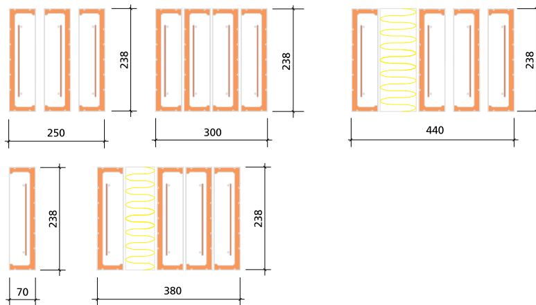
Przykłady ustawienia belek nadprożowych Porotherm 23.8 dla różnej grubości murów
