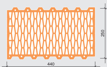
Przekrój pustaka Porotherm 44 Profi
