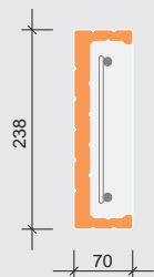
Przekrój belki nadprożowej 23.8
