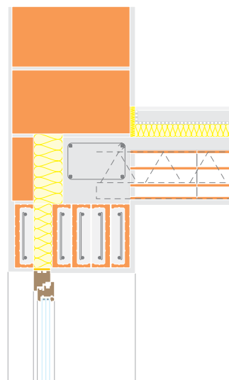
ściana Porotherm 44 P+W / EKO+ / Profi / Dryfix
