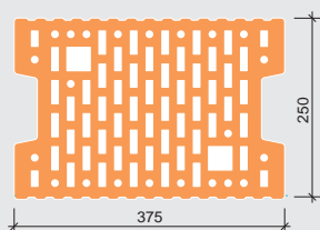
Przekrój pustaka Porotherm 25/37.5 AKU
