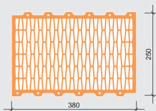
Przekrój pustaka Porotherm 38 Si
