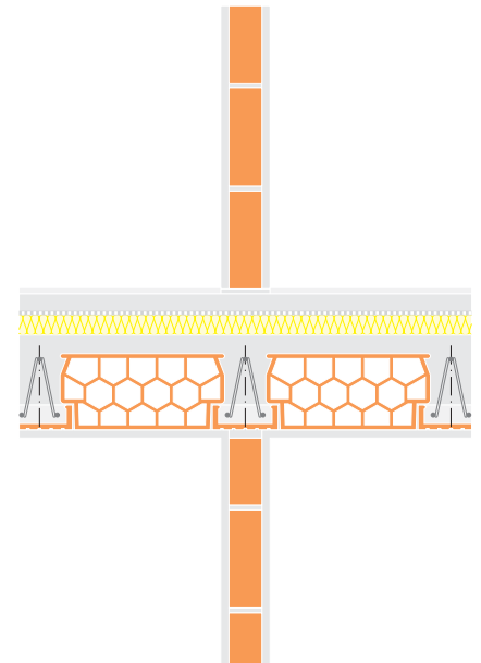
ściana Porotherm 8 P+W / Profi / Dryfix
