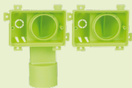
Puszka gniazda DYNAMIC: - z kolankiem bezpieczeństwa (CP032C) - na wprost (CP032D)
