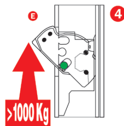
4. Dalsze obciążanie rygla: • powoduje zerwanie kołków C • obrót rygla do punktu E, rygiel jest dalej wysunięty z obudowy zamka • zamek pozostaje zamknięty Drzwi nie mogą zostać otwarte.
