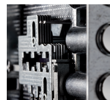
Zamek na klucz dwupiórowy ze specjalnym systemem zapadek.
