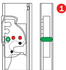
1. Zamek otwarty (drzwi otwarte)
