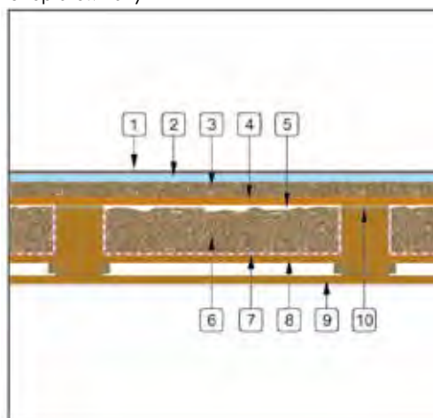
Strop drewniany
