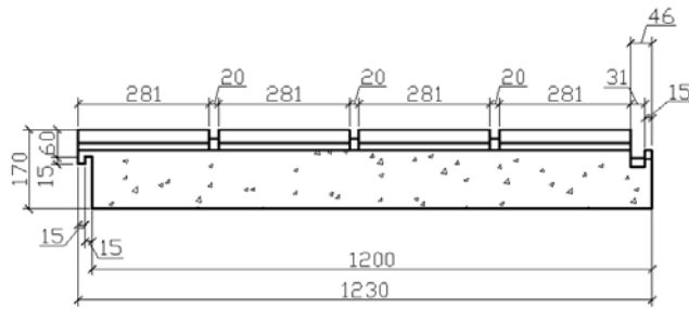
Systemu thermomur : element dachowy
