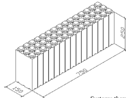
Systemu thermomur TH-400 : element ścienny dodatkowy
