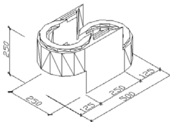
Systemu thermomur TH-250 : element ścienny dodatkowy
