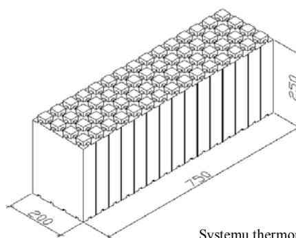
Systemu thermomur TH-400 : element ścienny wieńcowy
