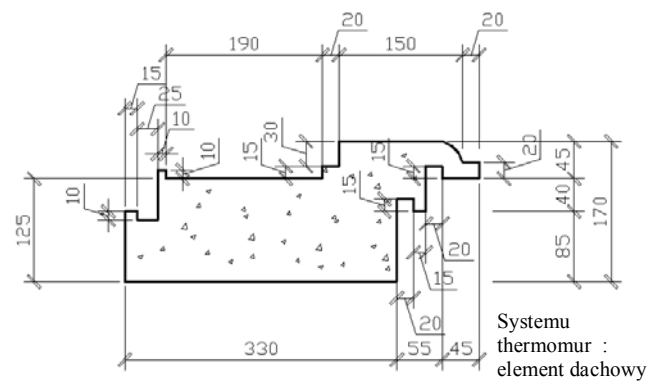
TH - 7 przekrój A-A
