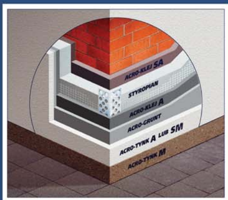
SCHEMAT SYSTEMU DOCIEPLEŃ
