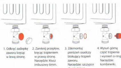
Fot. 2. Instrukcja wymiany o-ringów.
